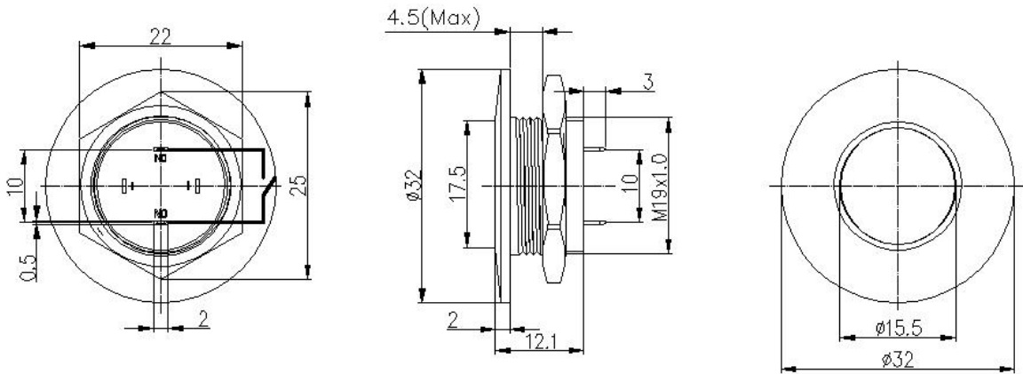
安装孔图
