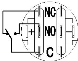
电气简图
