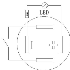
电气简图
